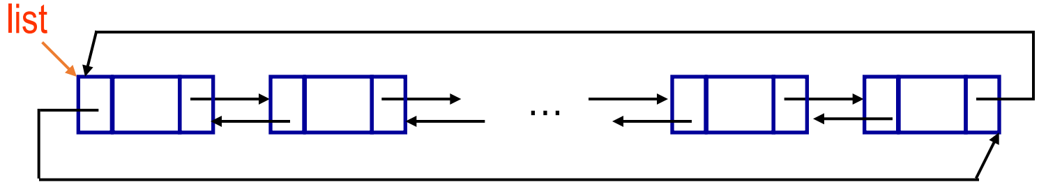
双向循环链表
