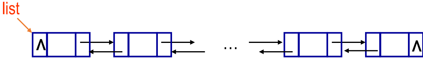
双向链表
